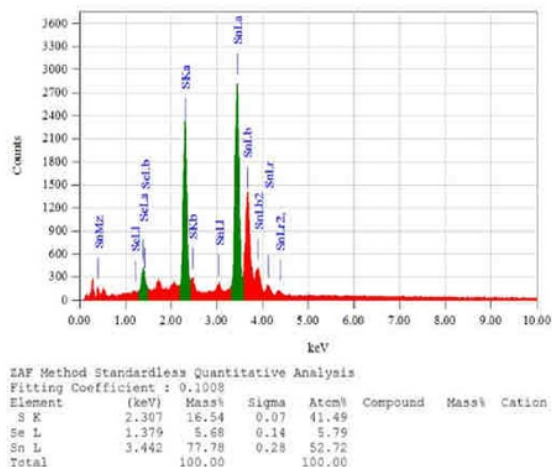
Gambar 6. Grafik antara intensitas dengan energi hasil karakterisasi EDAX lapisan tipis Sn(Se 0,2 S 0,8 ) dengan teknik evaporasi.
