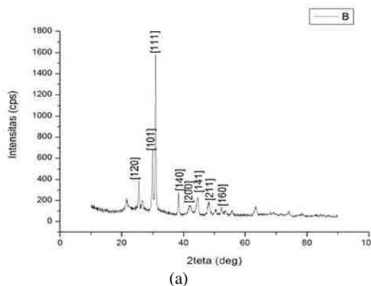
Gambar 2. Difraktogram XRD lapisan tipis Sn(Se 0,2 S 0,8 ) dengan spacer 25 cm
